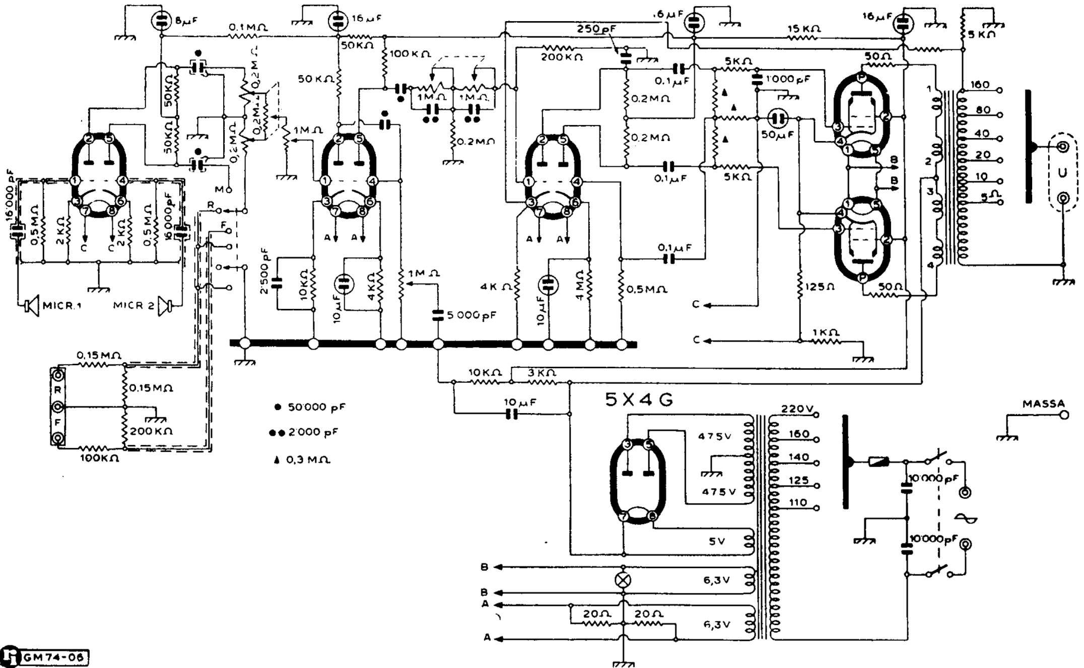
L.E.S.A. - Amplificatore mod. 535-T/2
